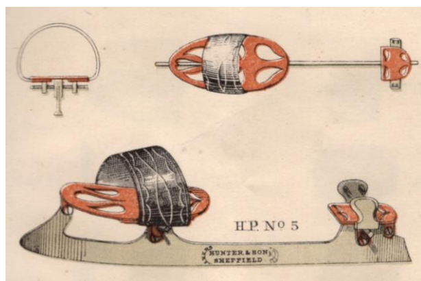
Afb.2 Hilliard's patent No. 5, damesschaats met voetkap die kan worden aangedraaid met de tweezijdige schroef.
