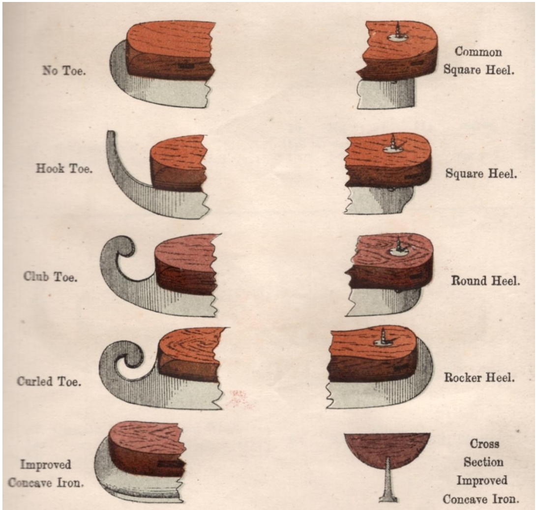
Afb. 3 Overzicht van uitvoeringsmogelijkheden aan de voor- en achterzijde van de schaatsen.
